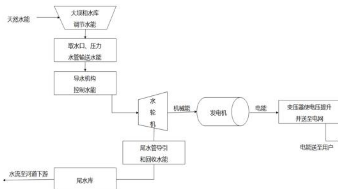
图 14-3：水力发电流程图
