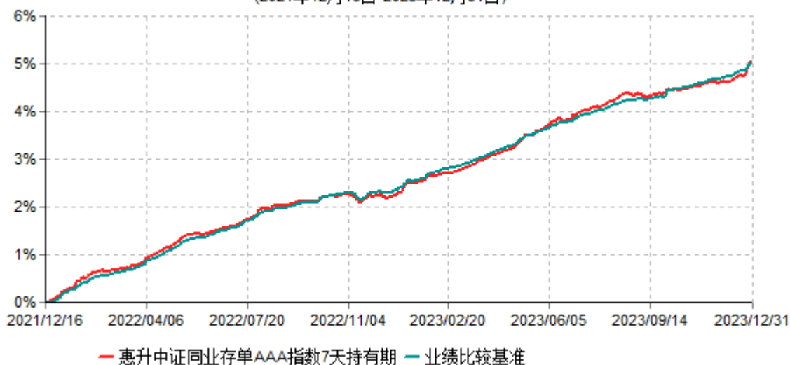
惠升中证同业存单AAA指数7天持有期证券投资基金累计净值增长率与业绩比较基准收益率历史走势对比图 (2021年12月16日-2023年12月31日)
