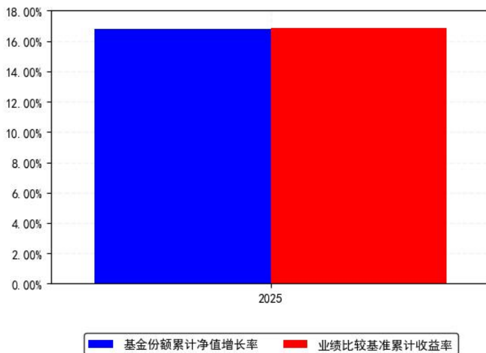
南方中证通用航空主题ETF每年净值增长率与同期业绩比较基准收益率的对比图
