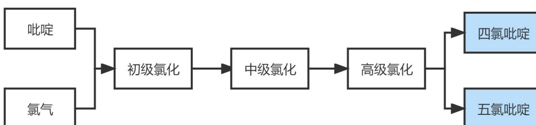
(2) 四氯吡啶和五氯吡啶的工艺流程图
