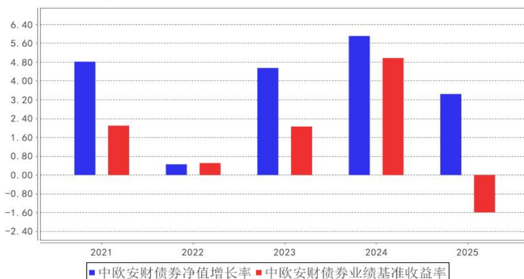
中欧安财债券基金每年净值增长率与同期业绩比较基准收益率的对比图
