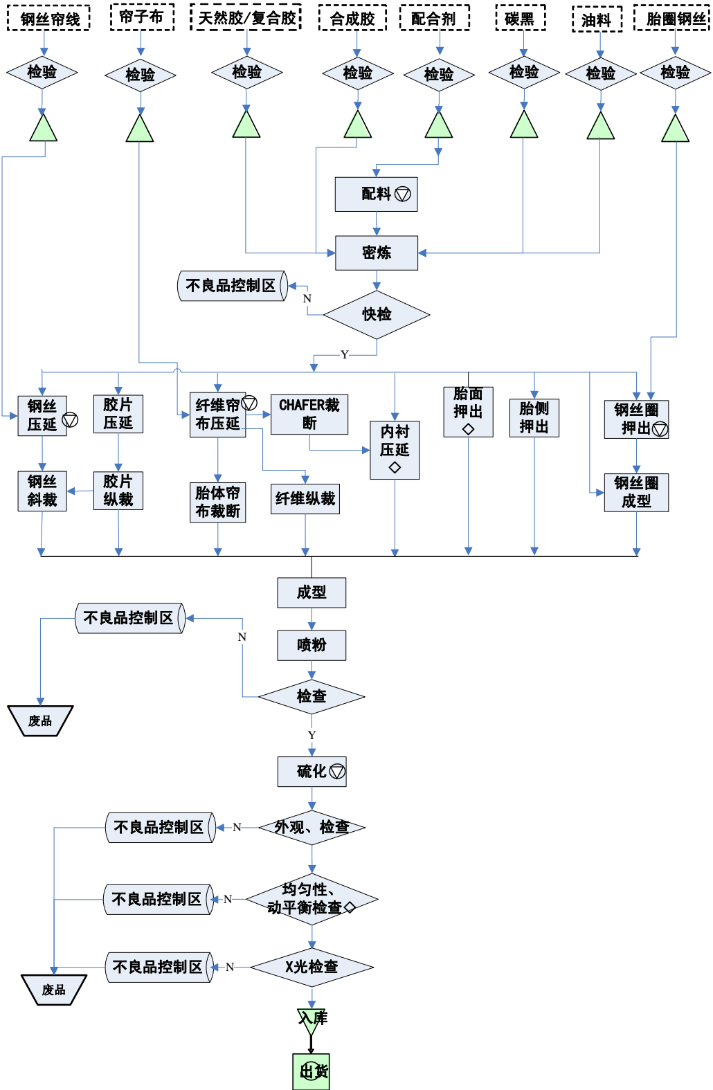
半钢子午胎生产工艺流程图：
