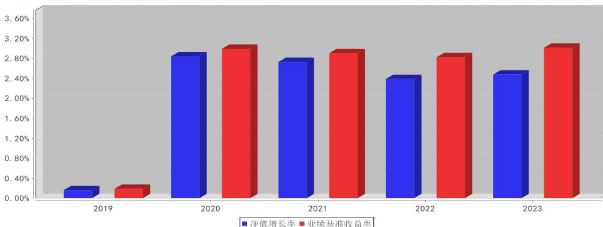
大成惠嘉一年定开债券A基金每年净值增长率与同期业绩比较基准收益率的对比图（2023年12月31日）
