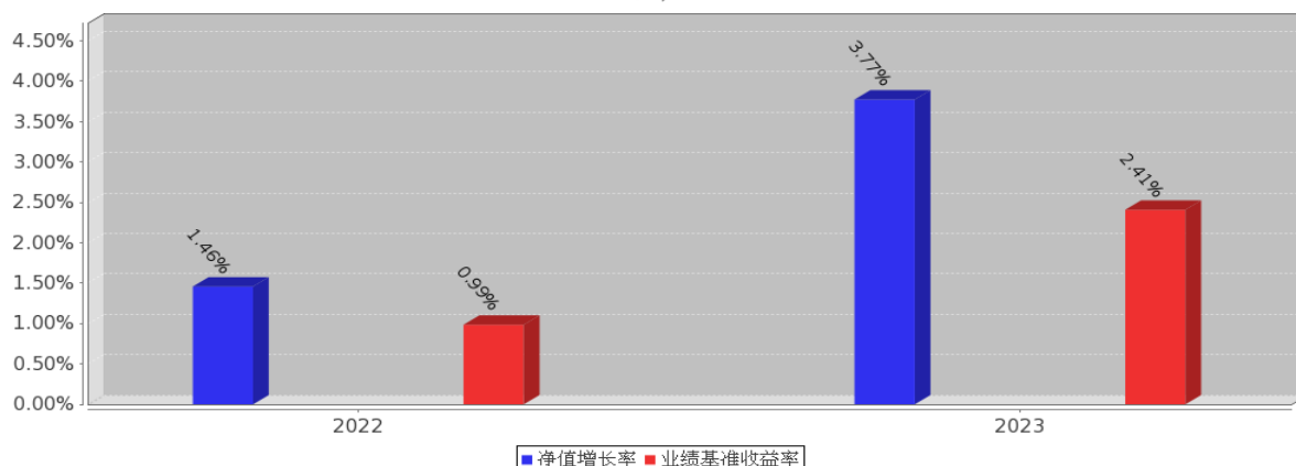
嘉实 90 天滚动持有短债 C 基金每年净值增长率与同期业绩比较基准收益率的对比图（2023 年 12 月 31 日）
