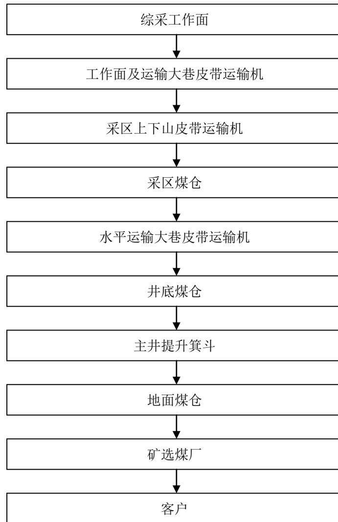
洗煤厂工艺流程图：
