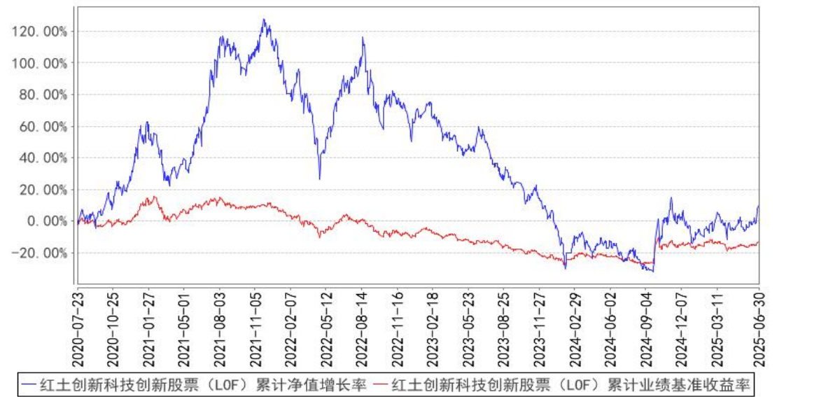
红土创新科技创新股票（LOF）累计净值增长率与同期业绩比较基准收益率的历史走势对比图
