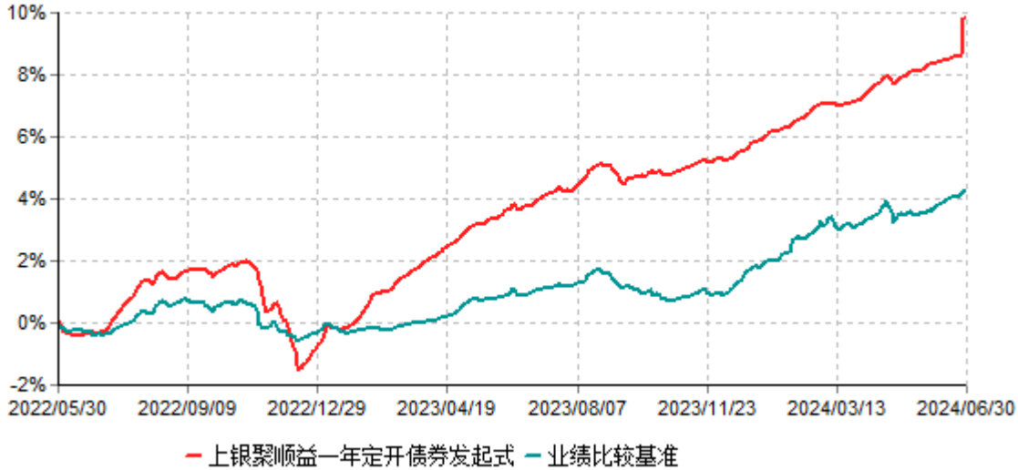
上银聚顺益一年定期开放债券型发起式证券投资基金累计净值增长率与业绩比较基准收益率 历史走势对比图 (2022年05月30日-2024年06月30日)
