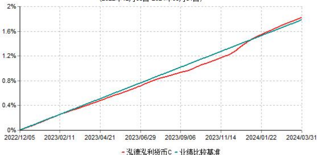
泓德泓利货币C累计净值收益率与业绩比较基准收益率历史走势对比图 (2022年12月05日-2024年03月31日)
