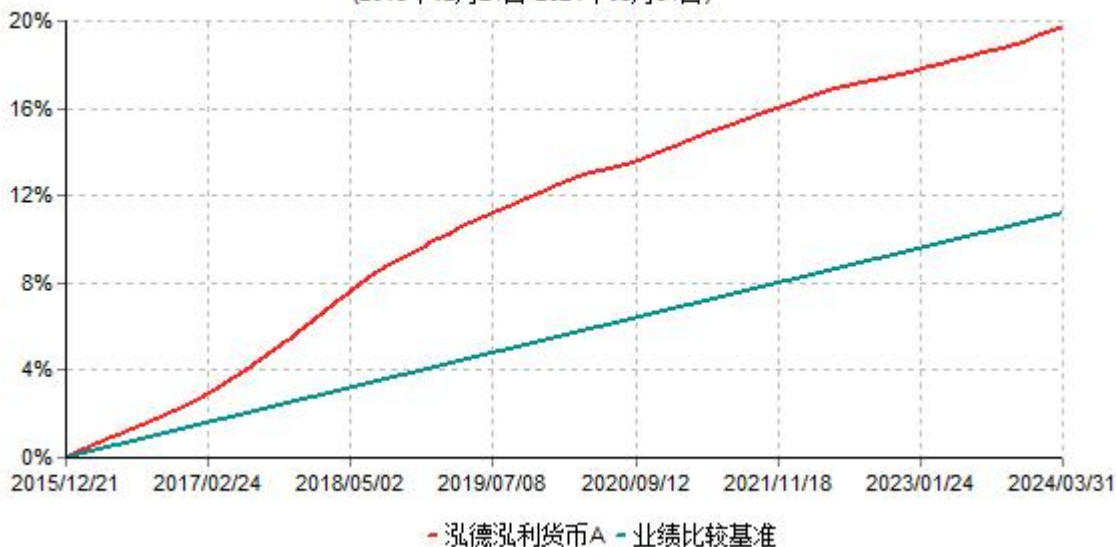
泓德泓利货币A累计净值收益率与业绩比较基准收益率历史走势对比图 (2015年12月21日-2024年03月31日)
