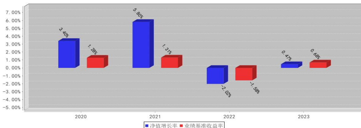
东方红招盈甄选一年持有混合A基金每年净值增长率与同期业绩比较基准收益率的对比图 (2023年12月31日)
