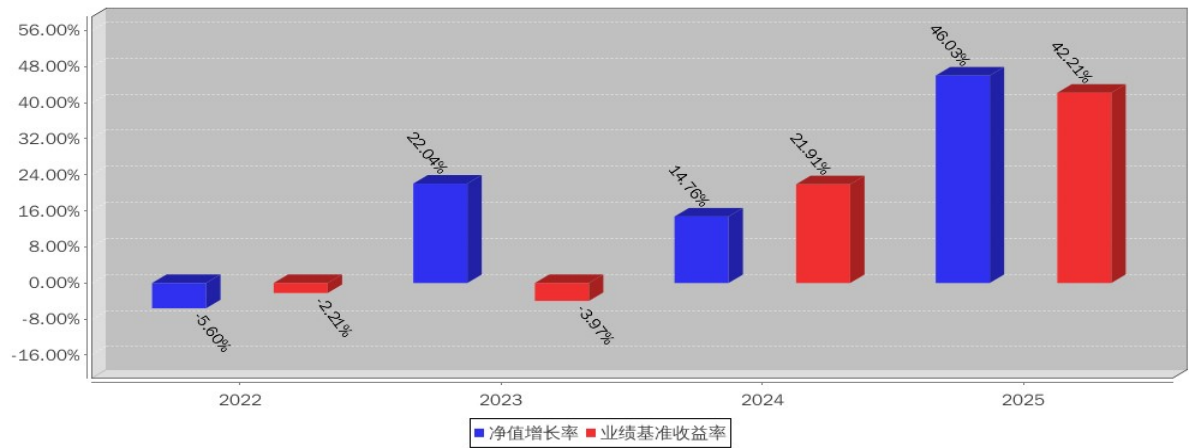
宝盈半导体产业混合发起式A基金每年净值增长率与同期业绩比较基准收益率的对比图（2025年12月31日）
