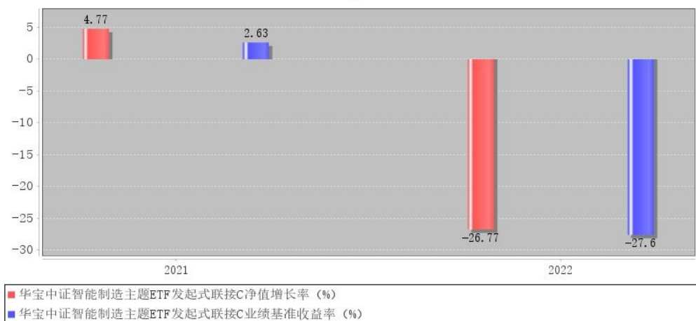
华宝中证智能制造主题ETF发起式联接C每年净值增长率与同期业绩比较基准收益率的对比图
