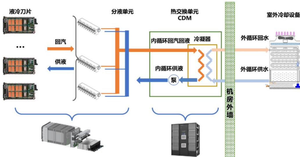
浸没相变液冷数据中心基础设施产品工作原理图
