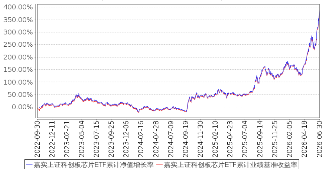
嘉实上证科创板芯片ETF累计净值增长率与同期业绩比较基准收益率的历史走势对比图 (2022年09月30日至2026年06月30日)
