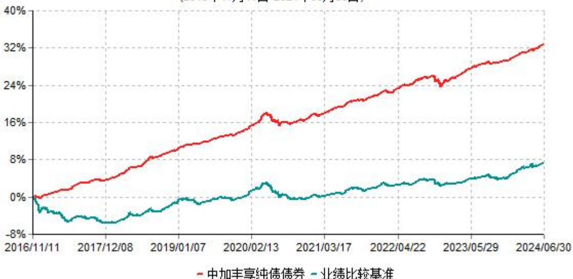
中加丰享纯债债券型证券投资基金累计净值增长率与业绩比较基准收益率历史走势对比图 (2016年11月11日-2024年06月30日)
