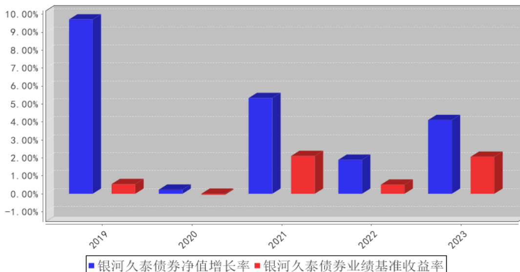
银河久泰债券基金每年净值增长率与同期业绩比较基准收益率的对比图
