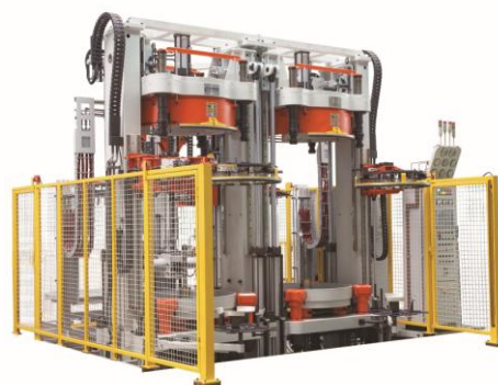
框架式硫化机和四柱式硫化机产品
