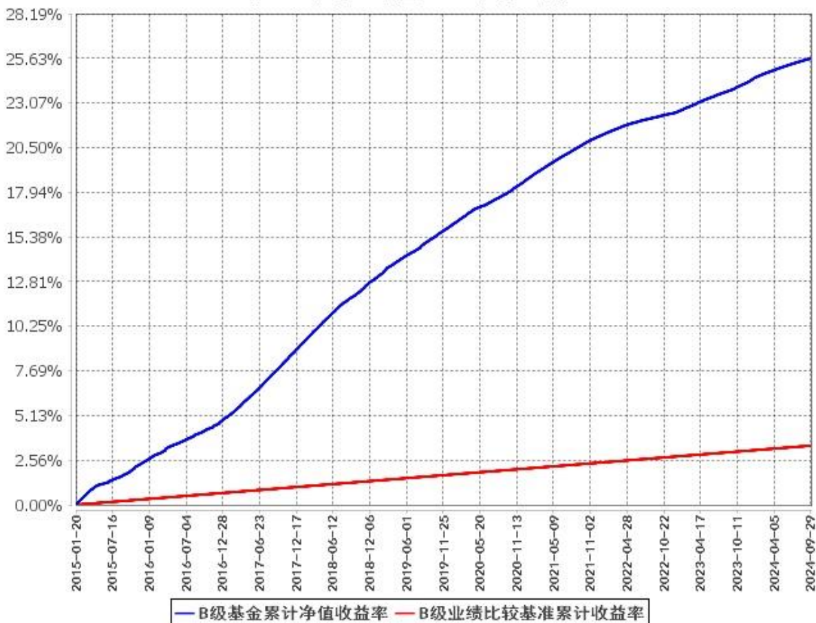
B级基金累计净值收益率与同期业绩比较基准收益率的历史走势对比图 (2015年1月20日至2024年9月30日)
