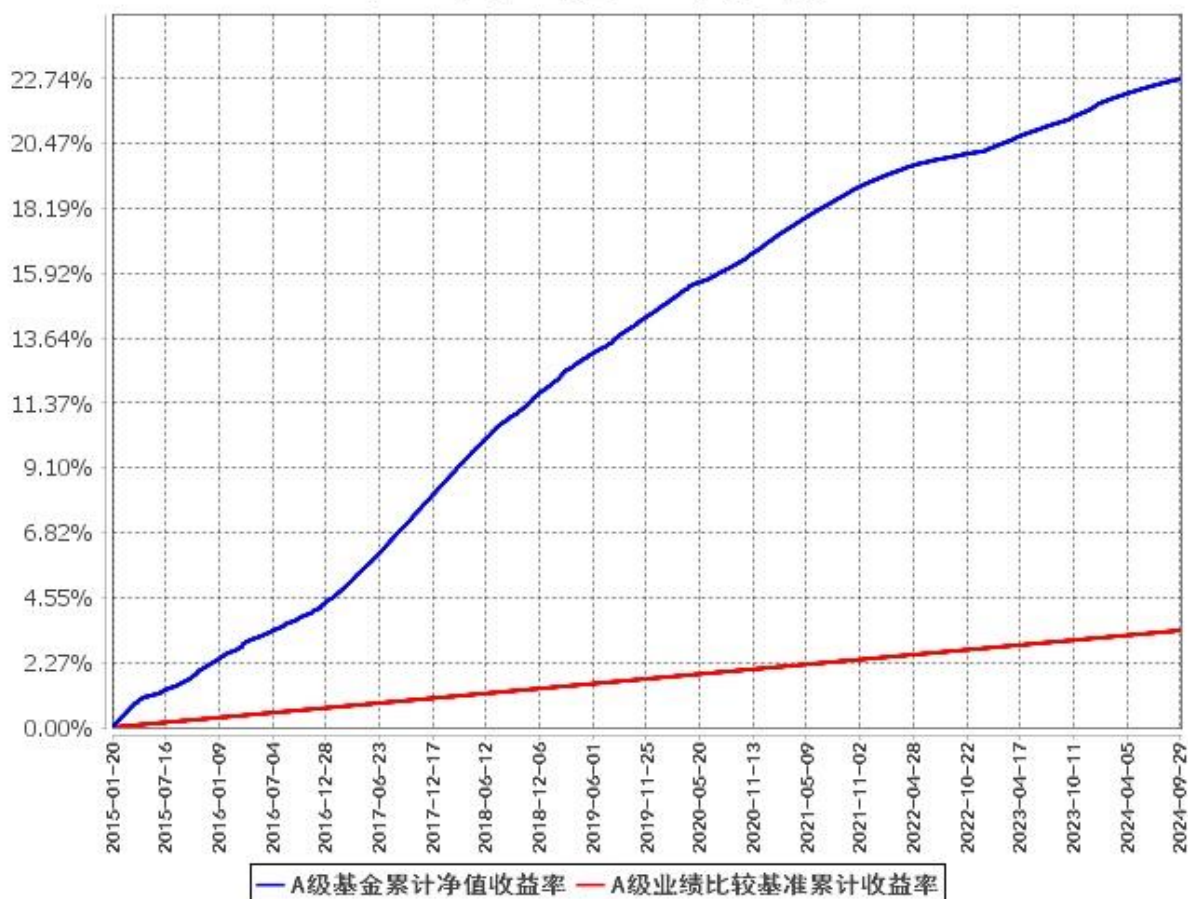
A级基金累计净值收益率与同期业绩比较基准收益率的历史走势对比图 (2015年1月20日至2024年9月30日)
