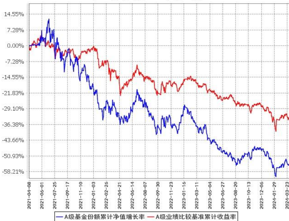
A级基金份额累计净值增长率与同期业绩比较基准收益率的历史走势对比图 (2021年4月8日至2024年3月31日)
