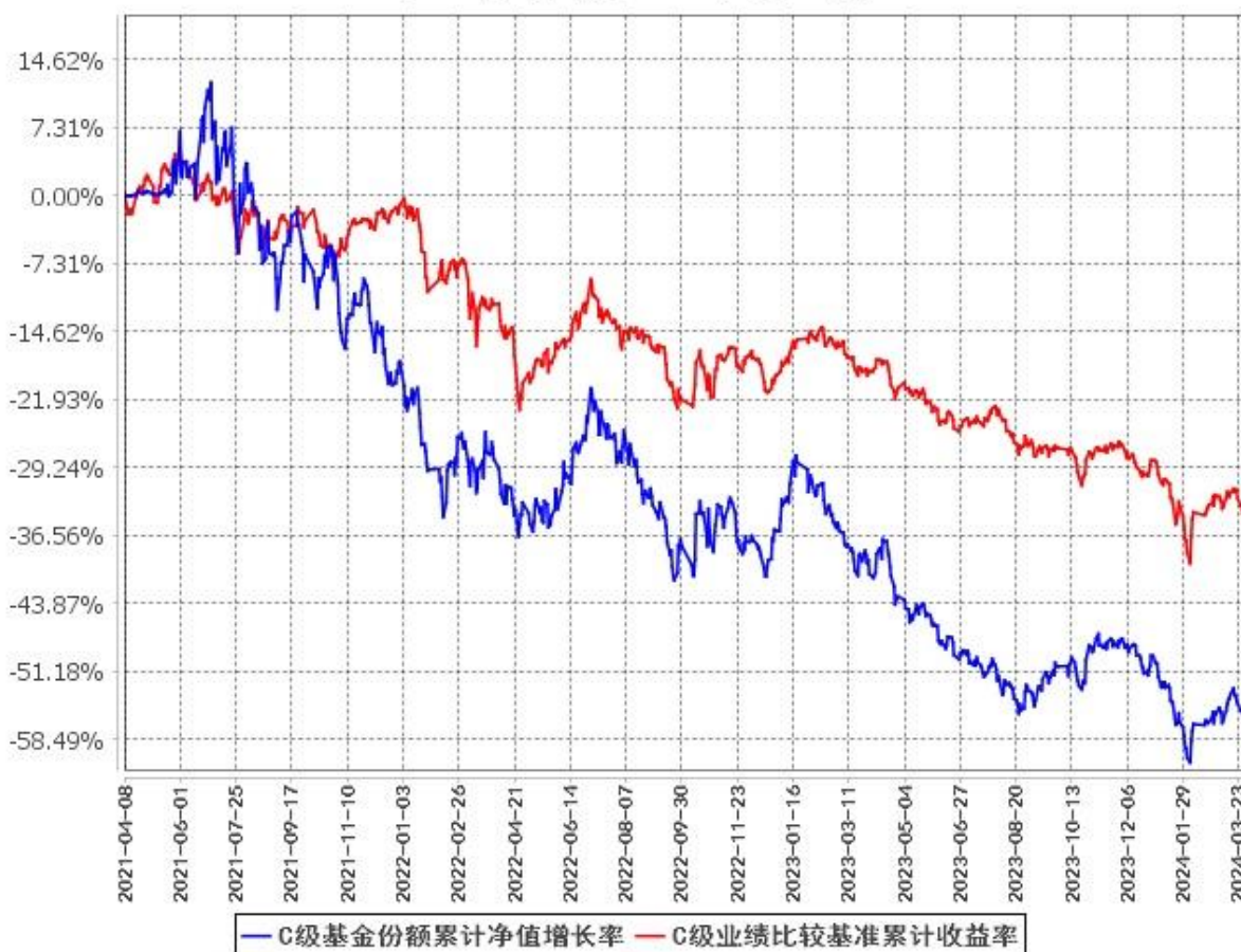
C级基金份额累计净值增长率与同期业绩比较基准收益率的历史走势对比图 (2021年4月8日至2024年3月31日)
