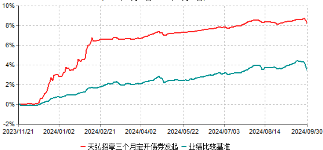
天弘招享三个月定期开放债券型发起式证券投资基金累计净值增长率与业绩比较基准收益率 历史走势对比图 (2023年11月21日-2024年09月30日)
