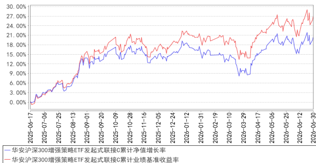
华安沪深300增强策略ETF发起式联接C累计净值增长率与同期业绩比较基准收益率的历史走势对比图
