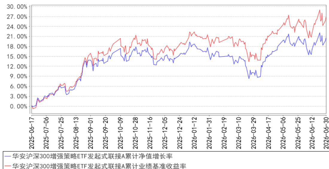
华安沪深300增强策略ETF发起式联接A累计净值增长率与同期业绩比较基准收益率的历史走势对比图
