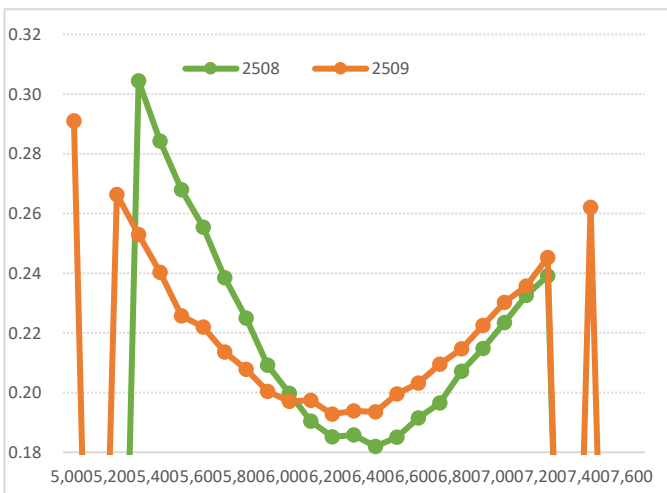
隐波率微笑
