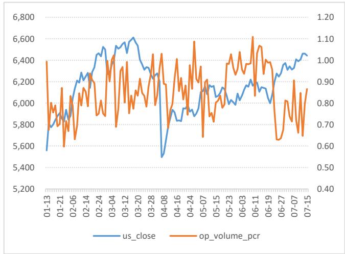
成交额-PCR
