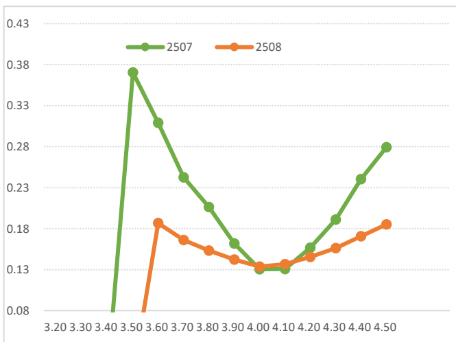
隐波率微笑
