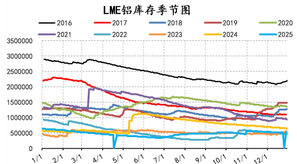
图 12：LME 铝库存
