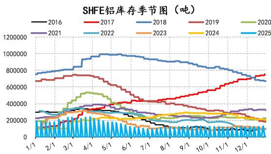
图 11：SHFE 铝库存
