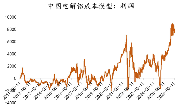
图 16：电解铝利润
