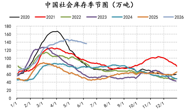
图 10：社会总库存
