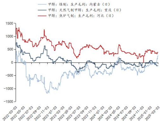
图8：三种工艺甲醇利润（元/吨）
