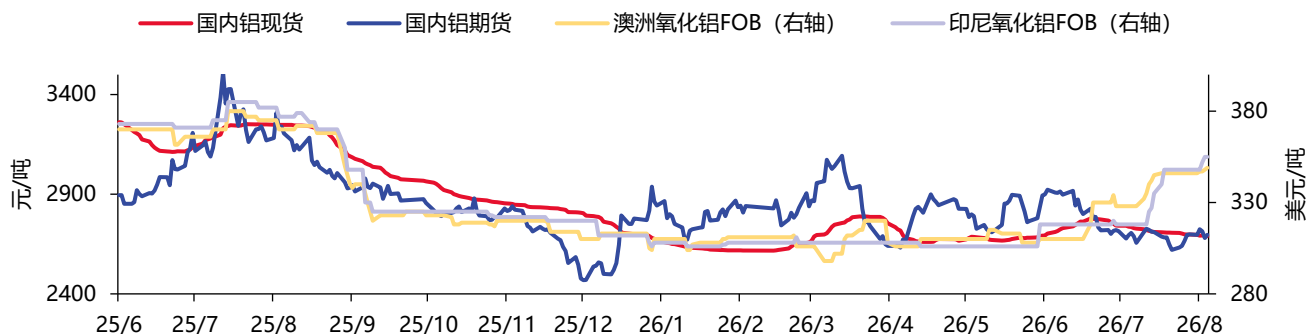
图表1：海内外氧化铝价
