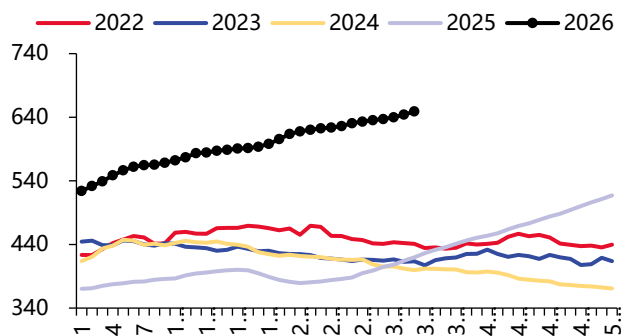
图表8: 氧化铝库存 (万吨)
