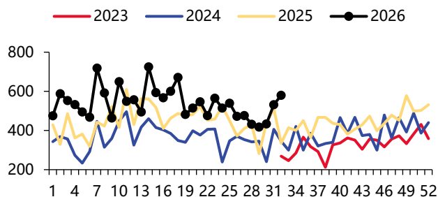
图表3: 铝土矿出港量 (万吨)
