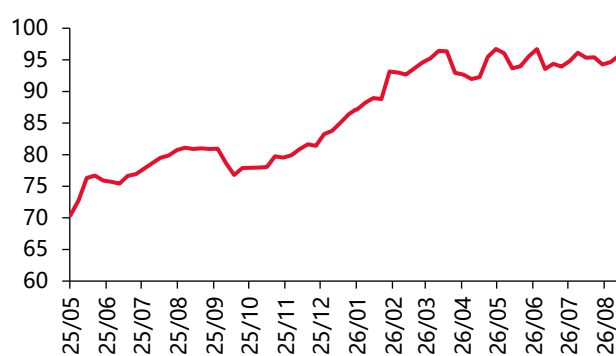
图表6: 铝土矿氧化铝厂库存天数 (天)
