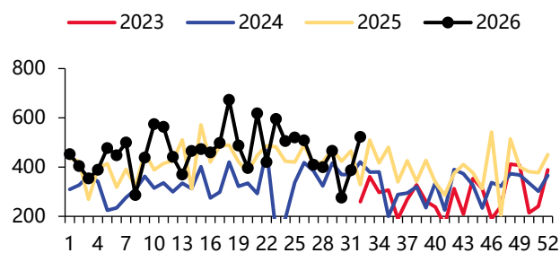
图表4: 铝土矿到港量 (万吨)
