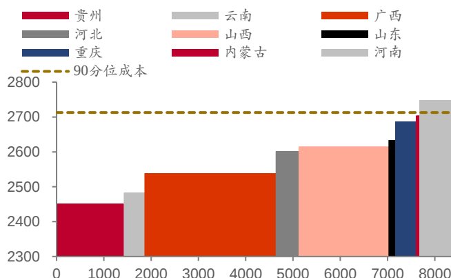
图表13: 氧化铝现金成本曲线 (元/吨)
