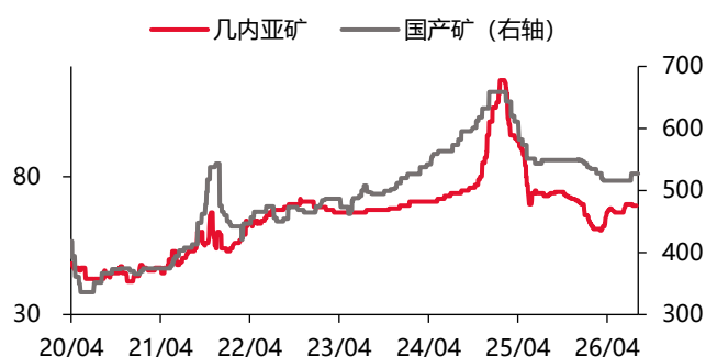
图表11: 海内外铝土矿价格 (美元/吨; 元/吨)
