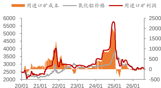
图表10: 氧化铝价格与即时盈利 (元/吨)
