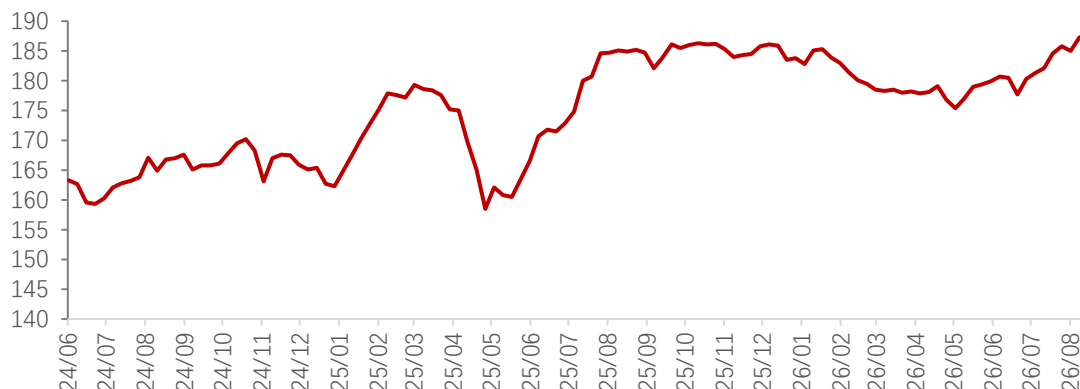
图表2：氧化铝产量 (万吨)
