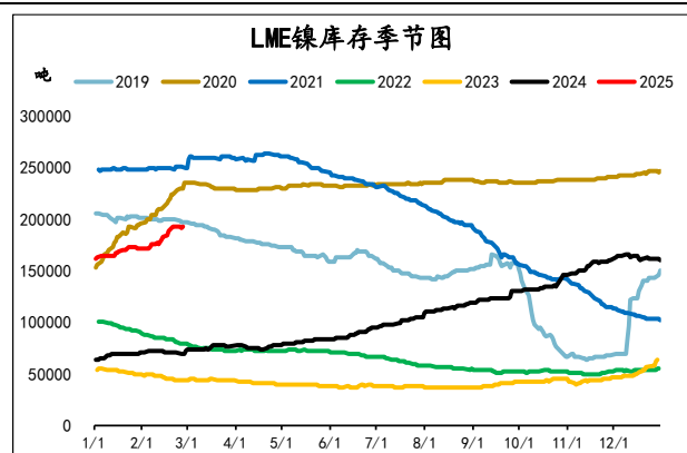
图 20. 镍 LME 库存
