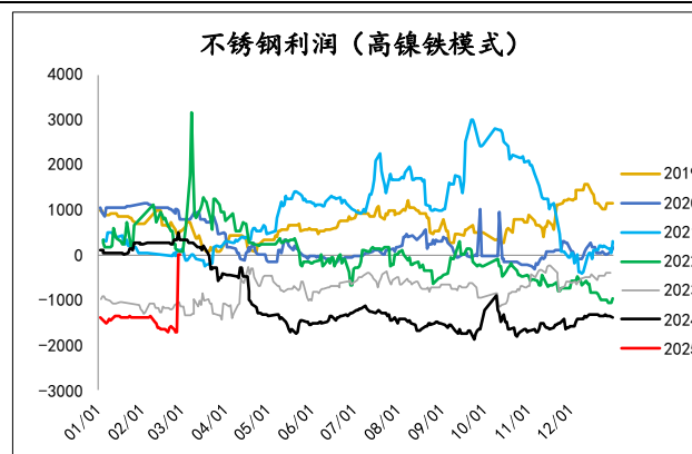
图 24. 不锈钢利润
