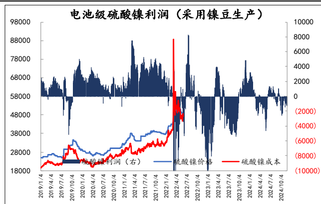
图 23. 硫酸镍利润
