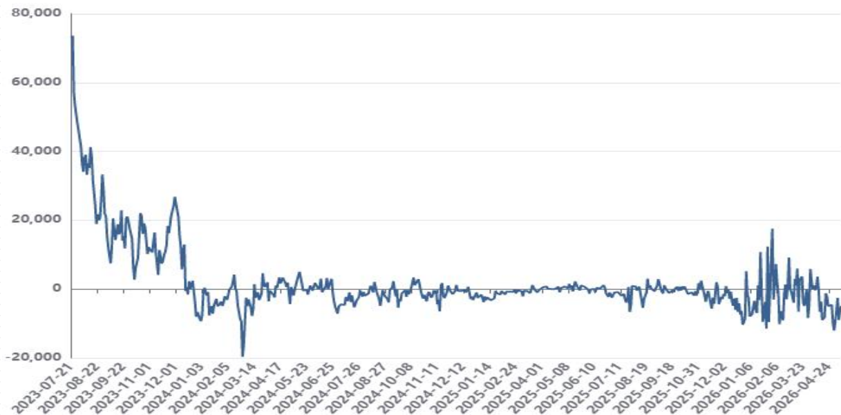
—●— 碳酸锂基差
