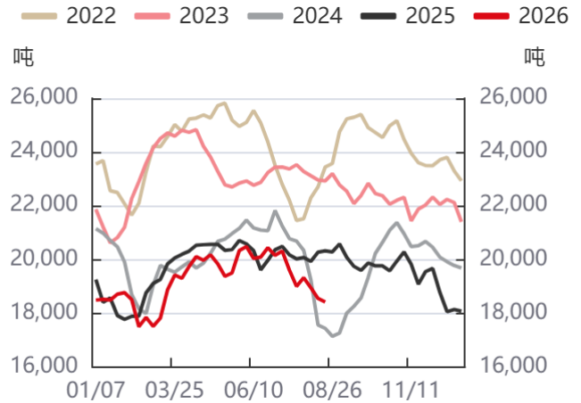
图12：硅铁：五大材需求量（周度）
