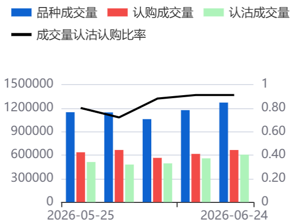
图6：日成交量(510300)
