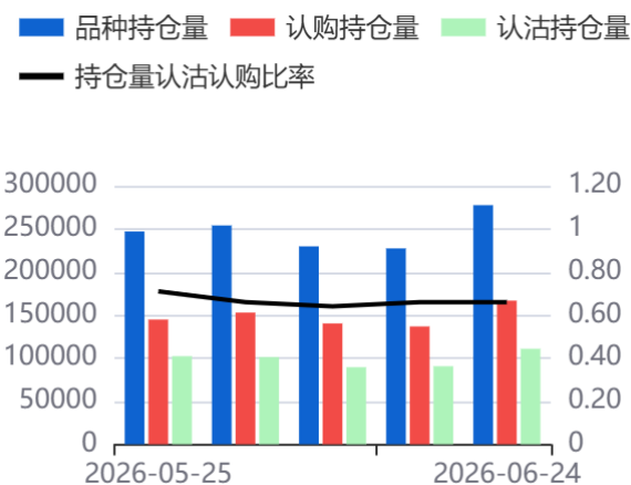
图12：日持仓量(159919)
