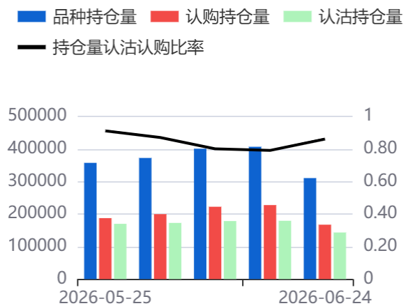
图22：日持仓量(000852)
