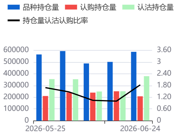
图57：日持仓量(588080)
