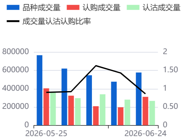
图56：日成交量(588080)
