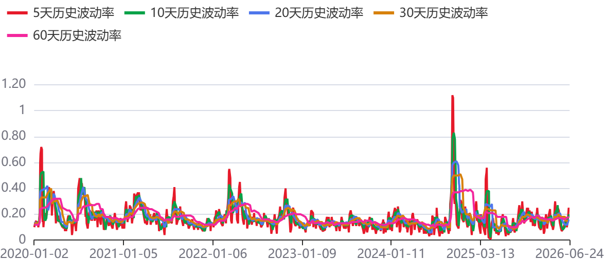
图8：历史波动率(510300)
