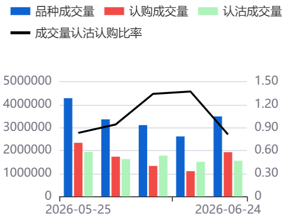
图51：日成交量(588000)
