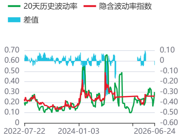
图25：波动率指数(000852)
