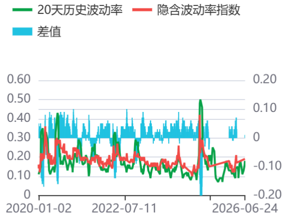
图5：波动率指数(510050)
