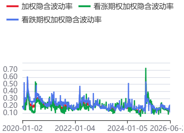
图19：隐含波动率(000300)
