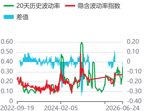
图30：波动率指数(510500)
