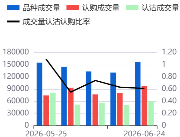
图11：日成交量(159919)
