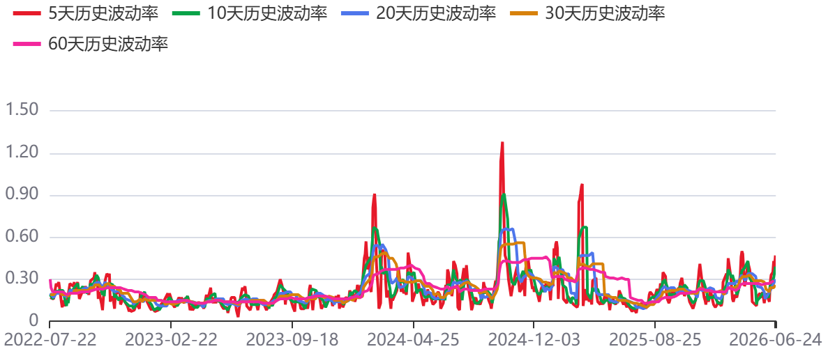
图23：历史波动率(000852)
