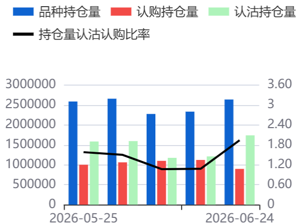
图52：日持仓量(588000)
