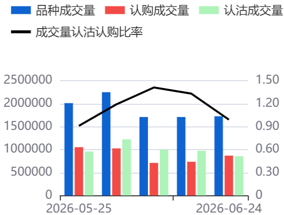
图26：日成交量(510500)
