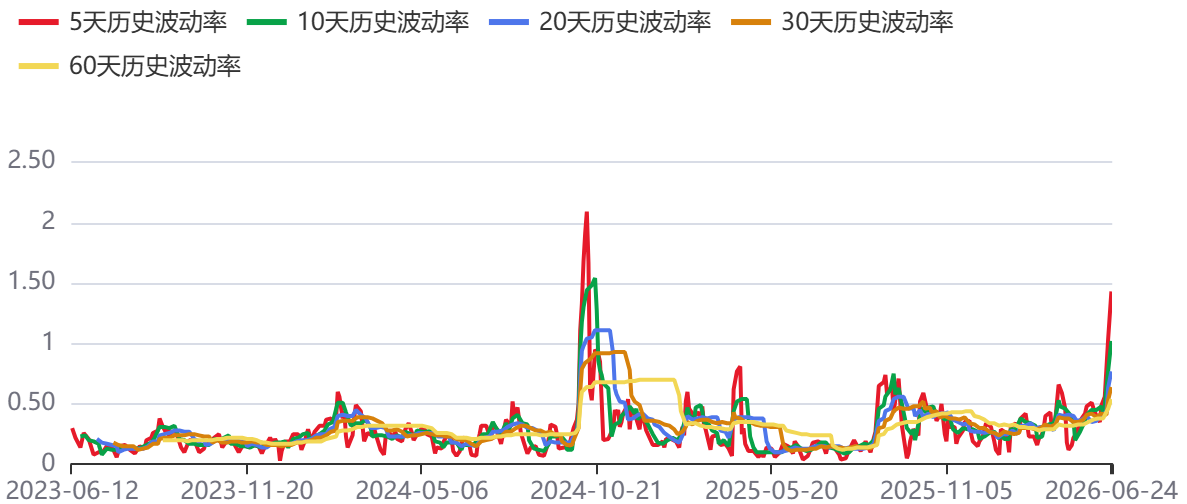
图58：历史波动率(588080)
