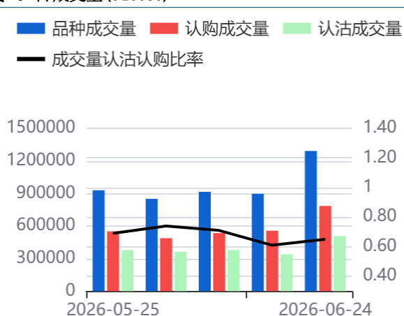
图1：日成交量(510050)
