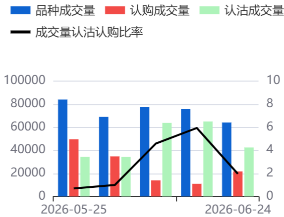
图41：日成交量 (159901)
