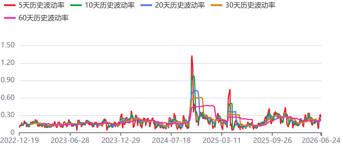
图43：历史波动率 (159901)
