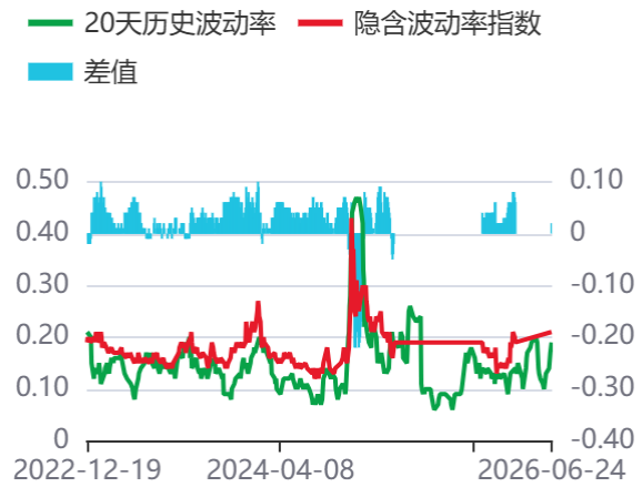
图50：波动率指数(000016)
