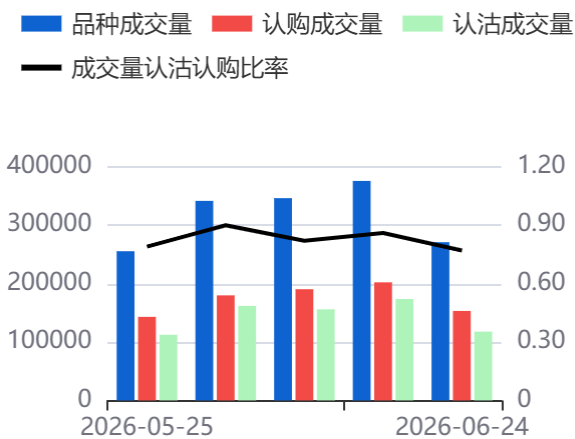
图21：日成交量(000852)
