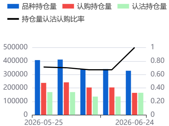
图37：日持仓量(159922)
