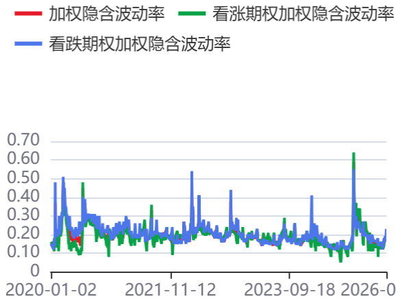
图4：隐含波动率(510050)
