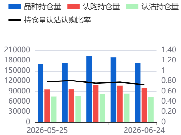
图17：日持仓量(000300)
