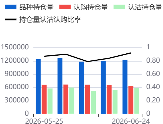
图7：日持仓量(510300)
