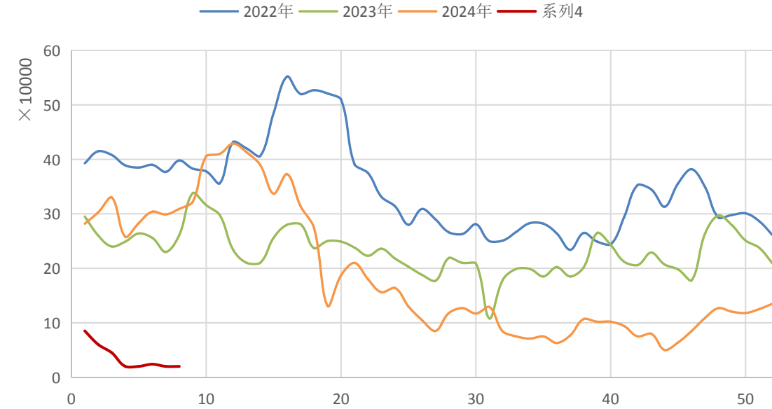
国内氧化铝港口库存：万吨
