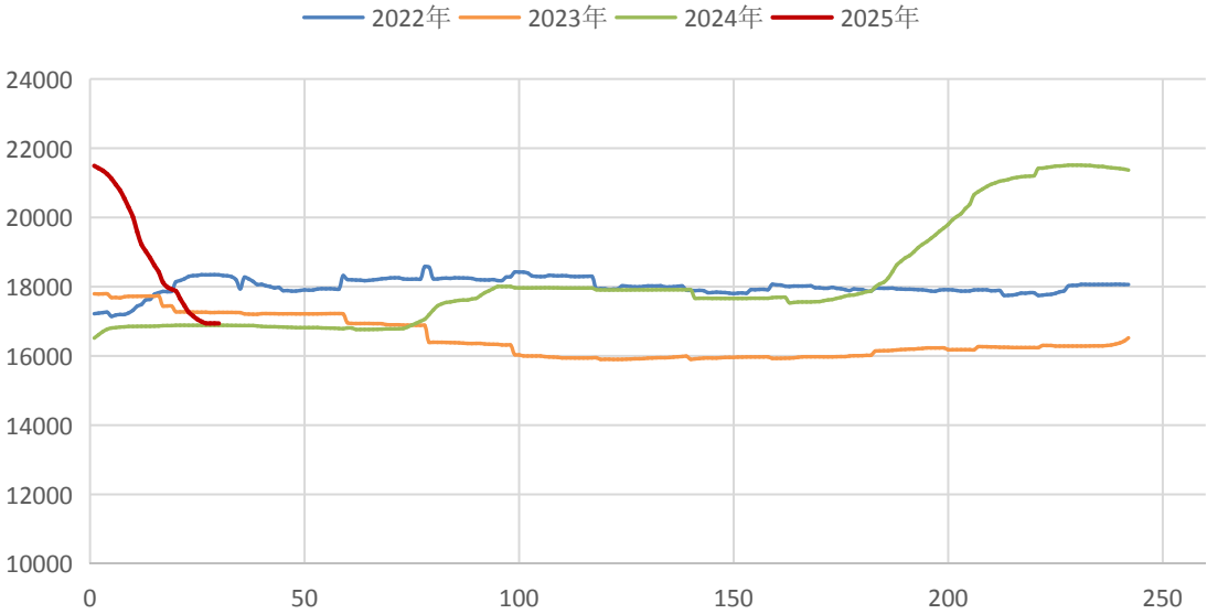
电解铝理论成本：元/吨
