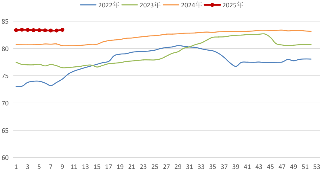
电解铝周度总产量：万吨
