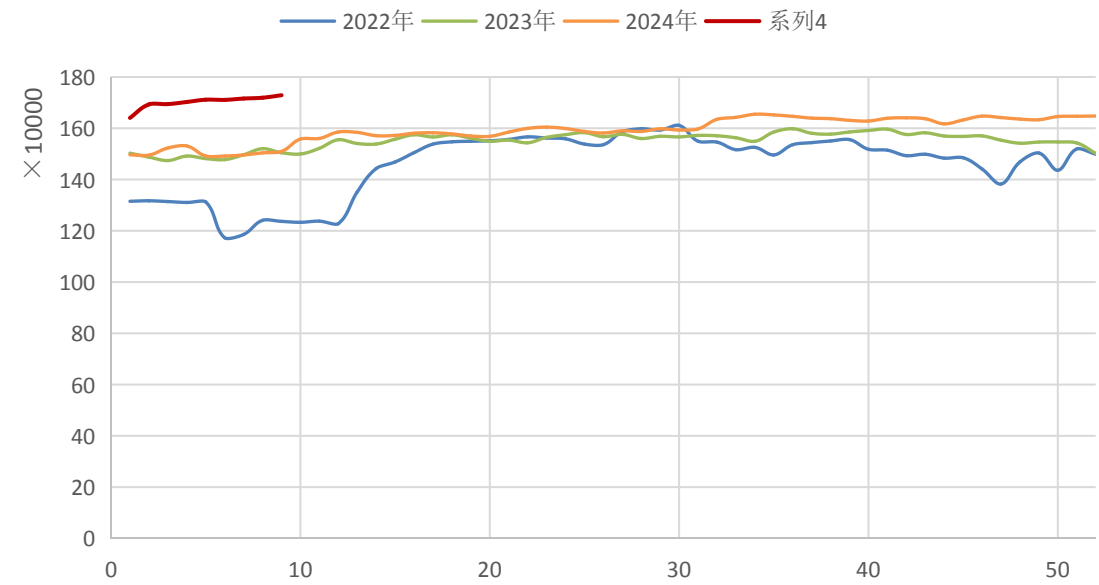
国内氧化铝周度产量：万吨
