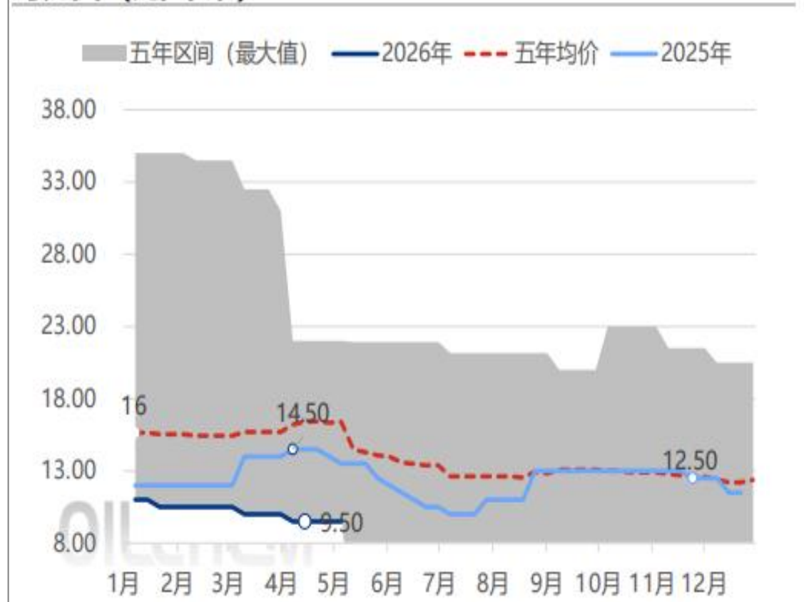
图2 2025-2026年光伏玻璃2.0mm单镀 (面板) 价格走势对比图 (元/平米)
