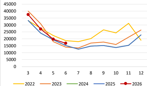
中型拖拉机产量（台）
