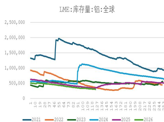
图5 LME库存
