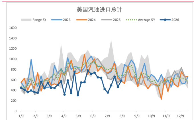
图表4：美国汽油进口总计（千桶/日）
