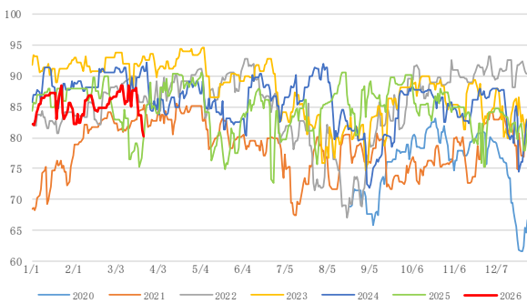
图 5： 纯碱开工率（%）
