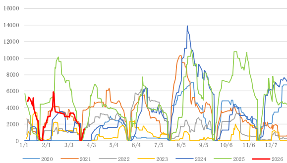
图 11： 纯碱仓单 (张)
