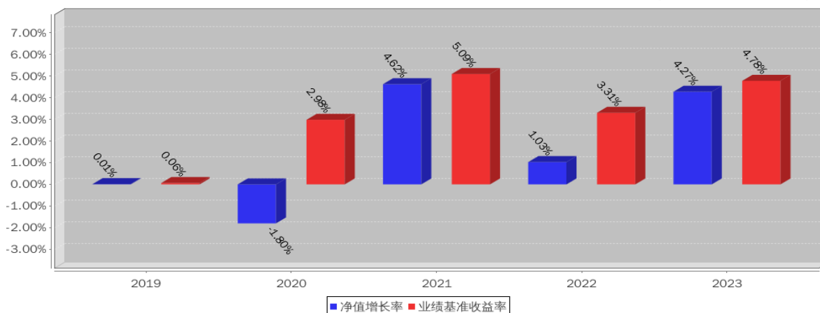
红塔红土瑞祥纯债债券C基金每年净值增长率与同期业绩比较基准收益率的对比图（2023年12月31日）
