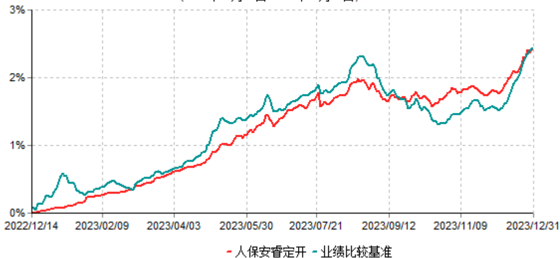
人保安睿一年定期开放债券型发起式证券投资基金累计净值增长率与业绩比较基准收益率历史走势对比图 (2022年12月14日-2023年12月31日)
