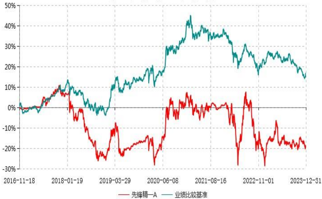
先锋精一A累计净值增长率与业绩比较基准收益率历史走势对比图 (2016年11月18日-2023年12月31日)
