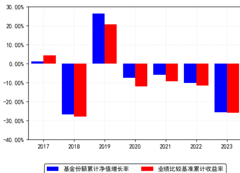
南方中证房地产ETF发起联接C每年净值增长率与同期业绩比较基准收益率的对比图（2023年12月31日）
