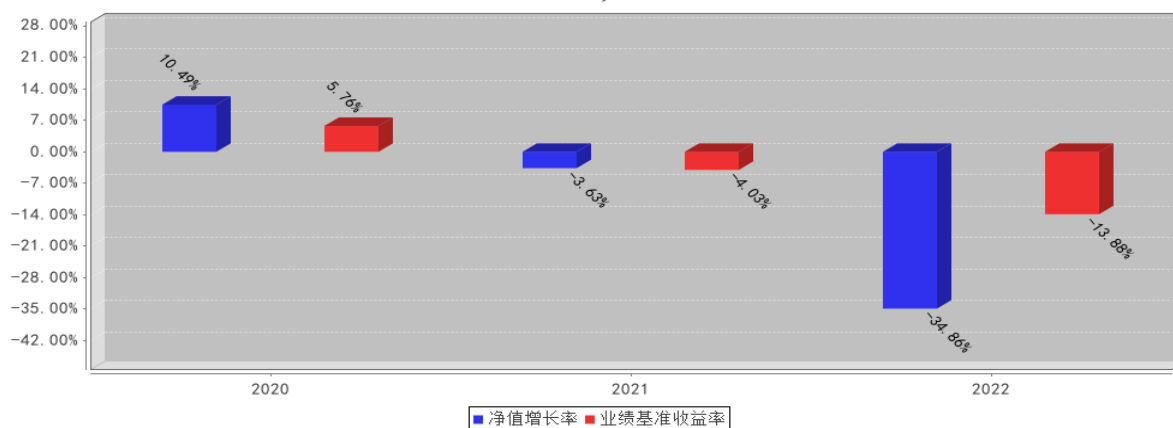
民生加银新动能一年定开混合C基金每年净值增长率与同期业绩比较基准收益率的对比图(2022年12月31日)
