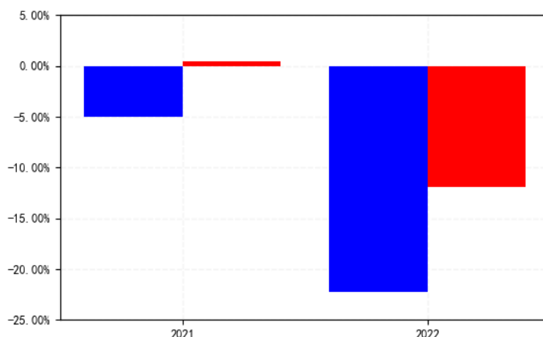
南方品质优选灵活配置混合C每年净值增长率与同期业绩比较基准收益率的对比图（2022年12月31日）
