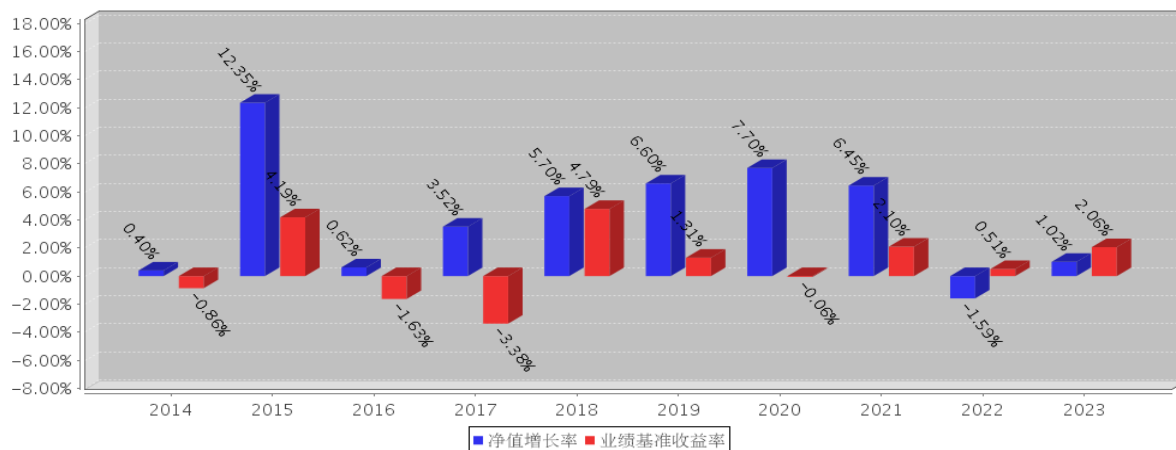
建信稳定得利债券A基金每年净值增长率与同期业绩比较基准收益率的对比图 (2023年12月31日)
